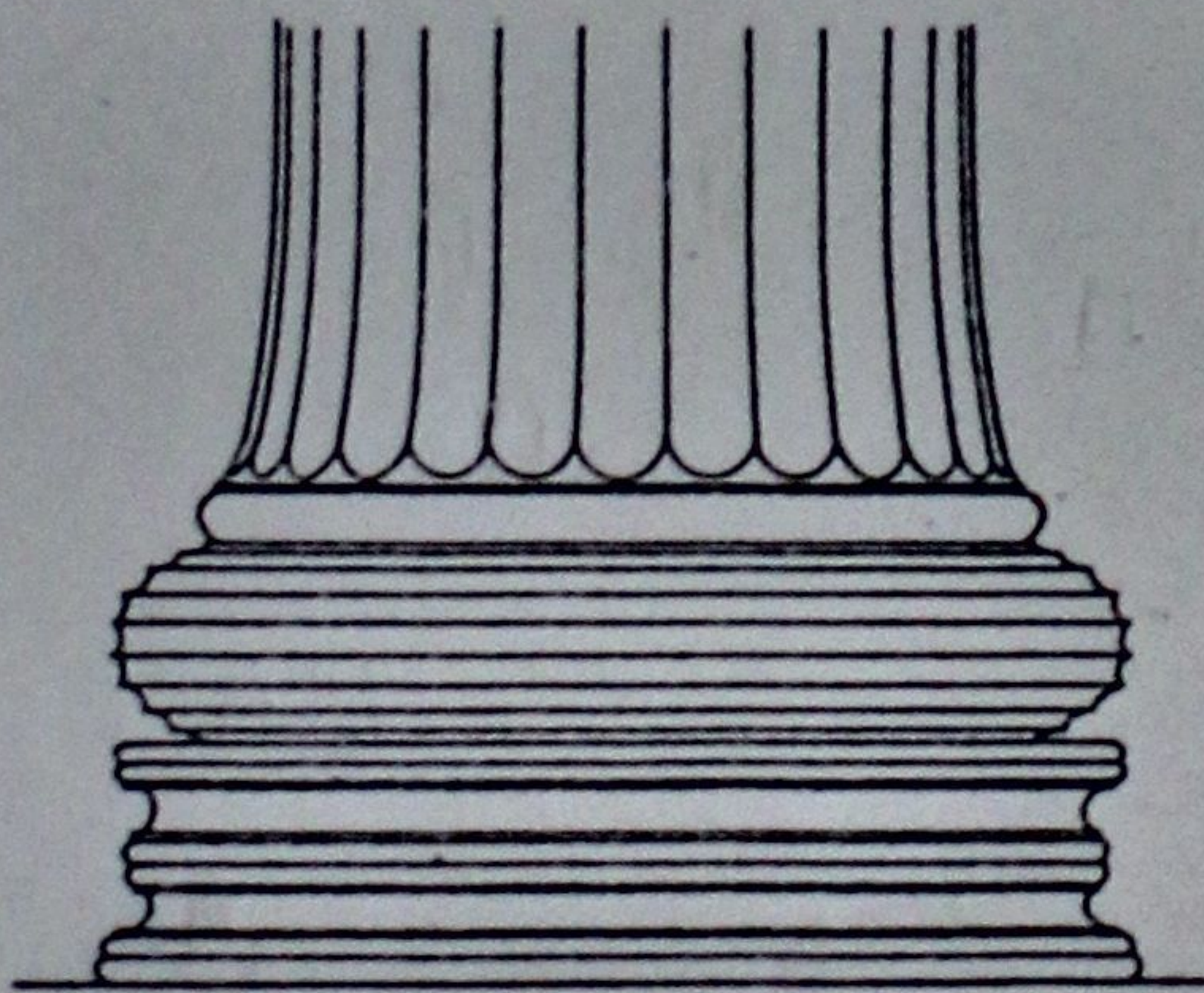
Εικ. 1. Βάση ιωνικού κίονα του ναού της Θέρμης. (Σχέδιο Ι. Τραυλιού).
