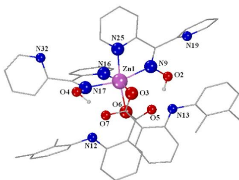
Σχήμα 23: Κρυσταλλική δομή [Zn(Mef)_2(Hrko)_2]
