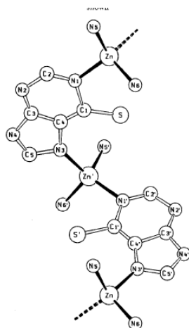
Σχήμα 7 : Κρυσταλλική δομή του συμπλόκου [Zn(Mer)(NH 3 ) 2 ] \cdot H 2 O
